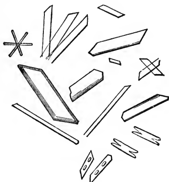
Fig. 2.—INOSITE.
